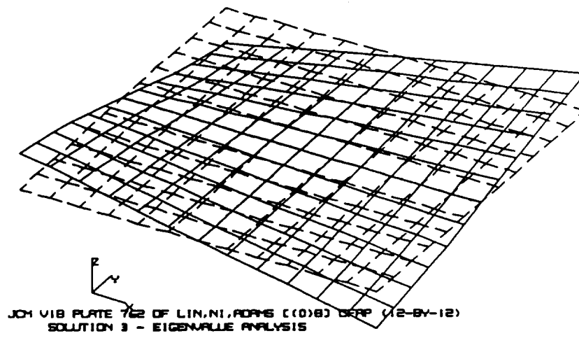
Fig. 8a. Plate 762, Mode 1
