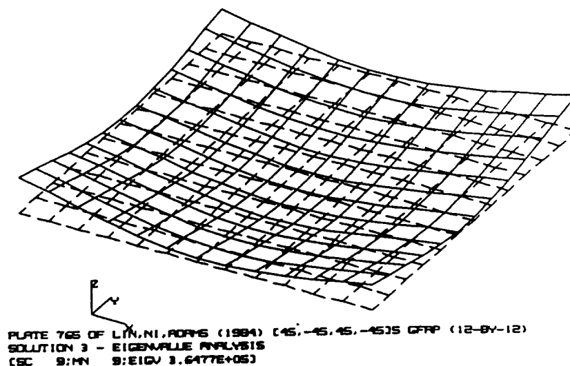
Fig. 5c. Plate 765, Mode 3
