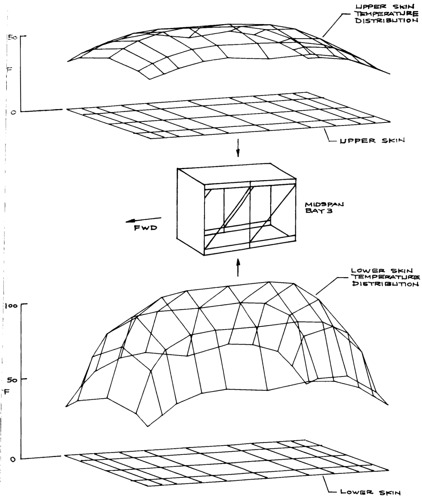
(d) SPAR thermal model D.
