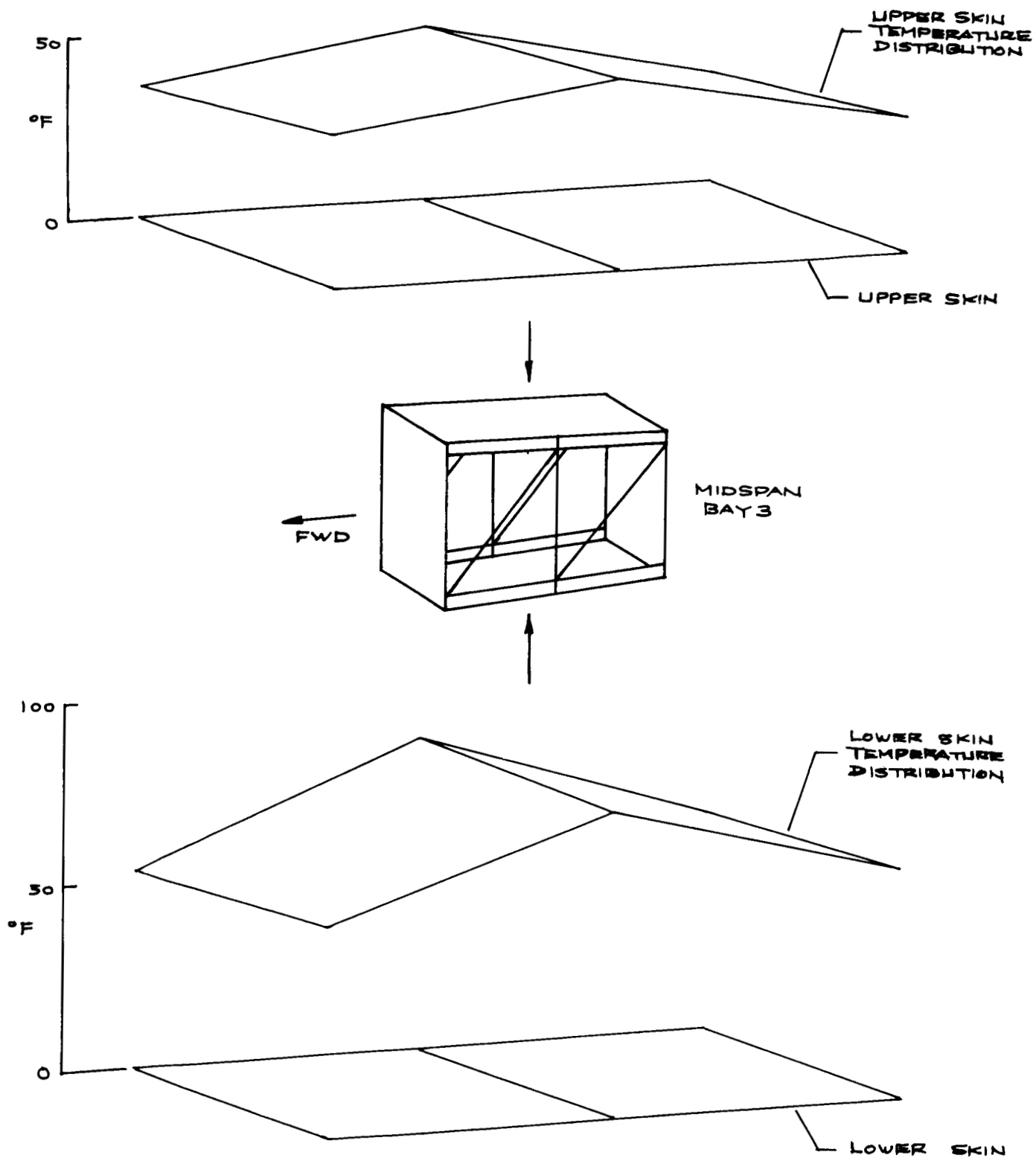
(a) SPAR thermal model A.
