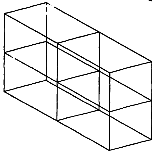
4 IHEX2 Elements
